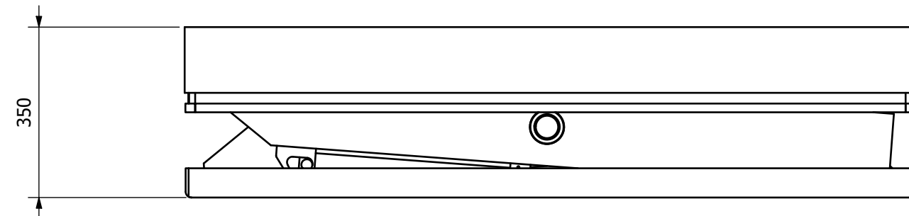
Lock ( 1 : 11 )
