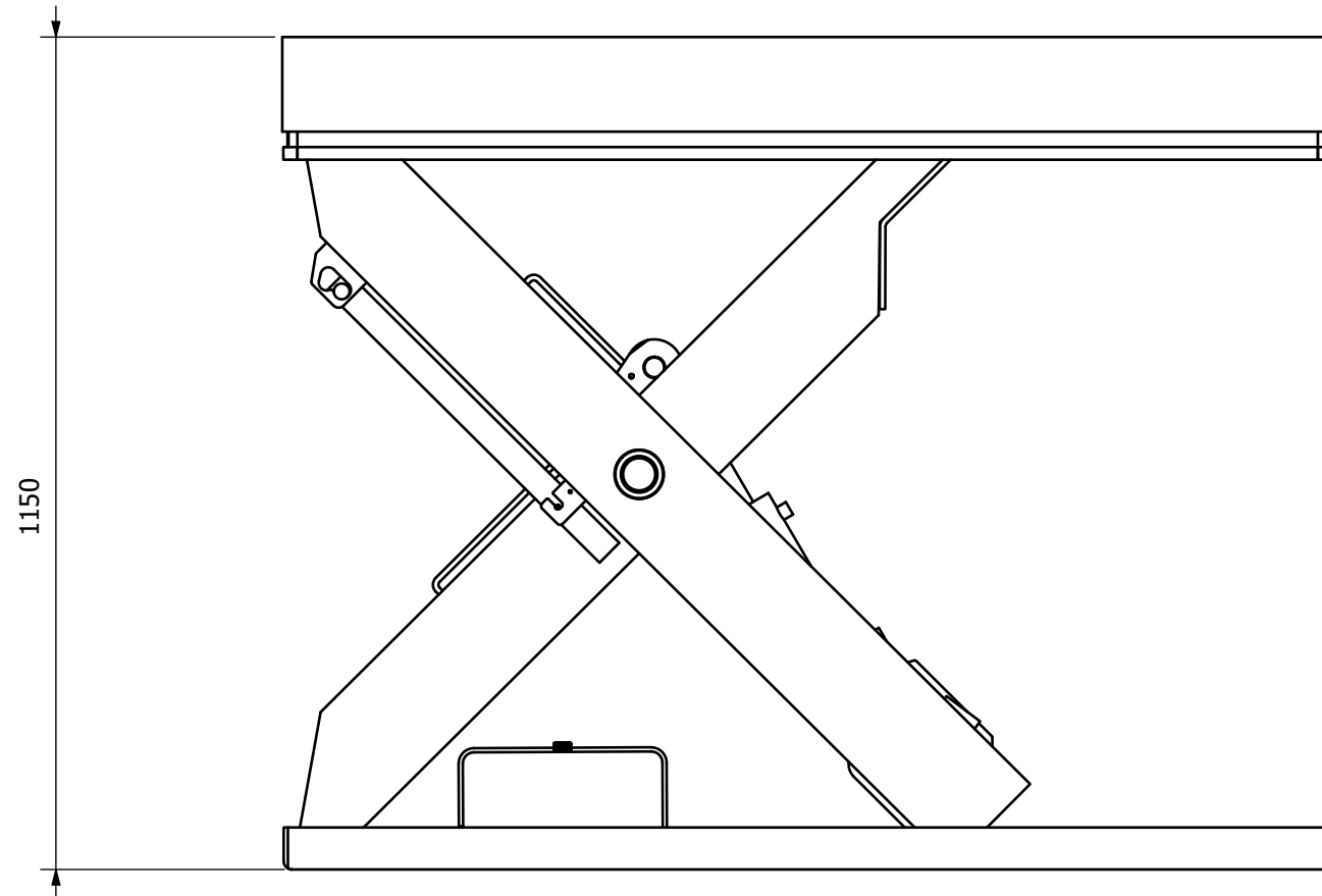
Overløft ( 1 : 11 )
