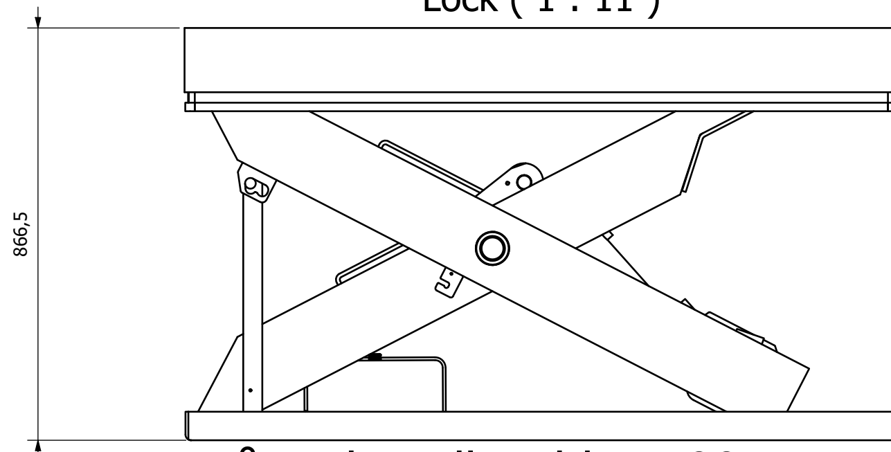
Lock ( 1 : 11 )
