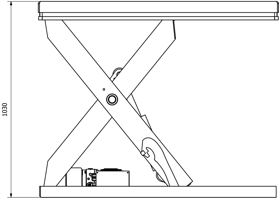
BH ( 1 : 10 )
