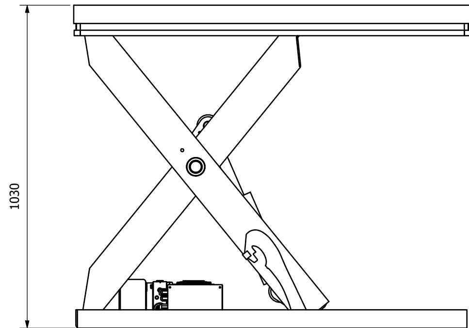
Overløft ( 1 : 12 )
