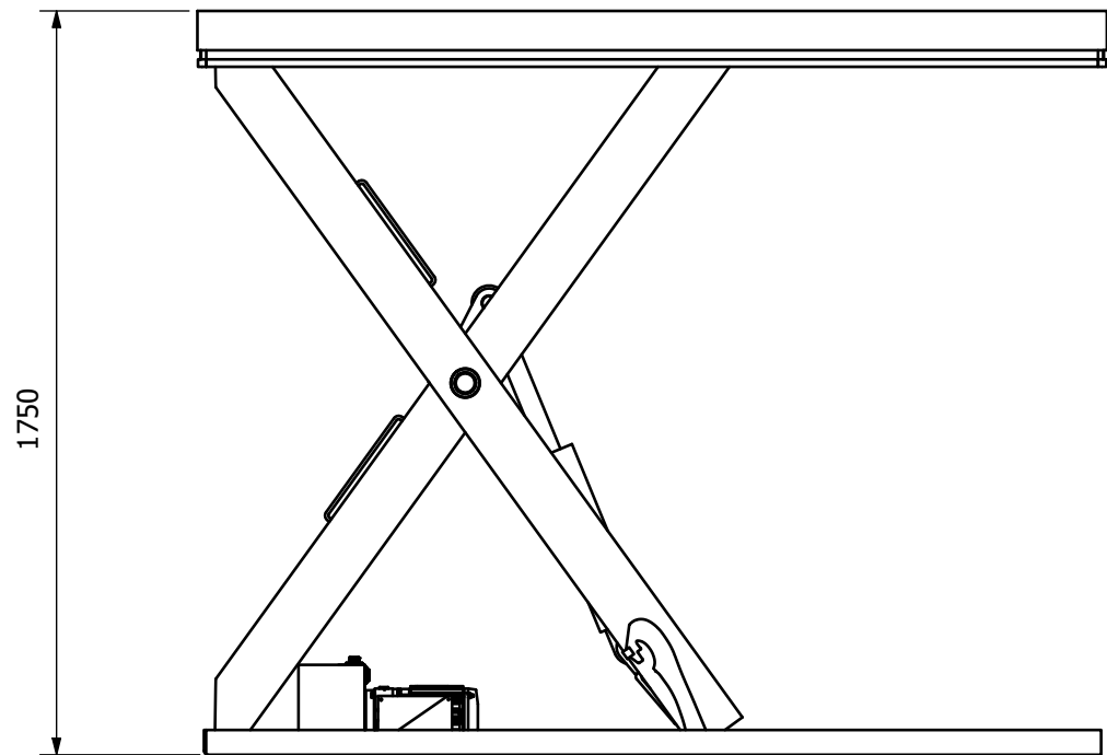
Overløft ( 1 : 20 )
