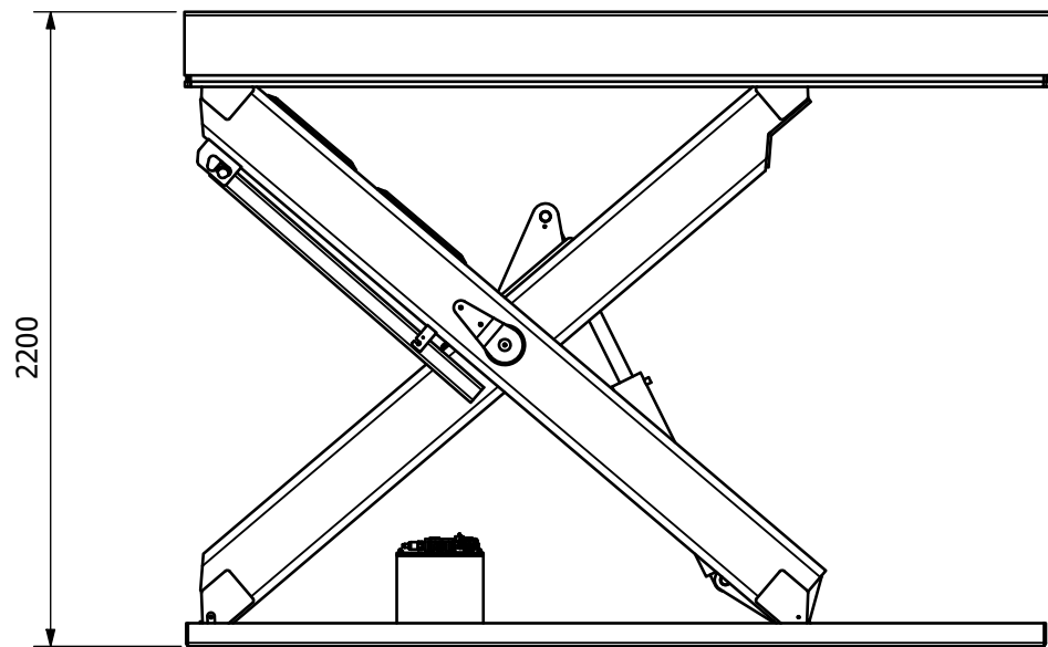
TOP ( 1 : 29 )
