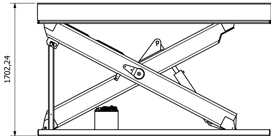
SERVICE ( 1 : 29 )
